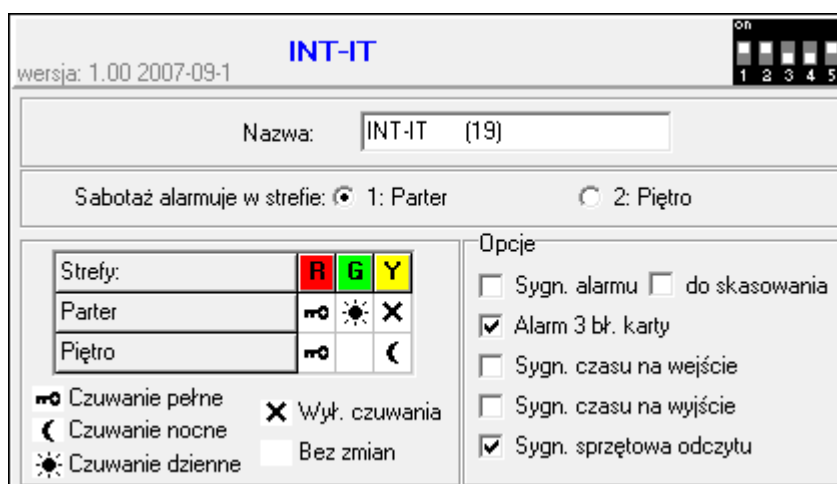
Rys. 16. Programowanie ustawień modułu sterowania strefami w programie DLOADX (przykładowa konfiguracja).
