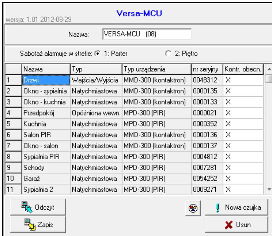
Rys. 15. Programowanie ustawień kontrolera systemu bezprzewodowego 433 MHz oraz czujek bezprzewodowych 433 MHz w programie DLOADX (przykładowa konfiguracja).
