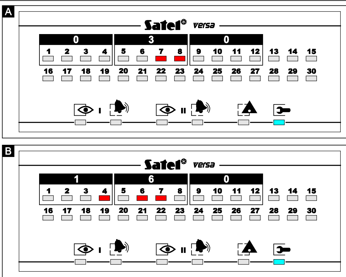
Rys. 1. Przykłady prezentowania wartości dziesiętnych przy pomocy diod LED w manipulatorze LED. W przykładzie A zaprogramowana jest wartość 30 (030), a w przykładzie B – 160.
